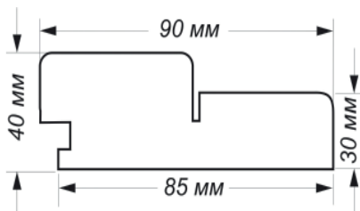
КОРОБКА 40*90
