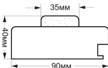
КОРОБКА МАЯТНИКОВАЯ
