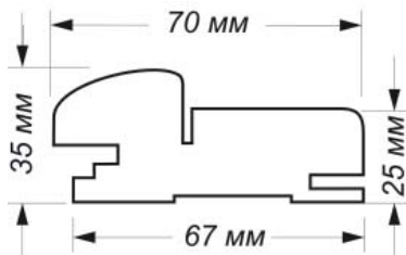
КОРОБКА СТАНДАРТНАЯ 35*70
