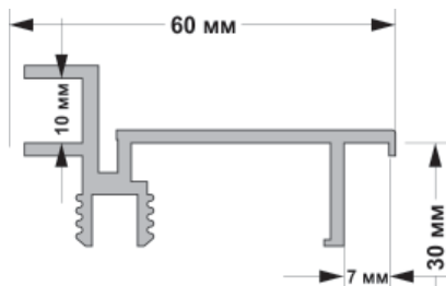
КОРОБКА АЛЮМИНИЕВАЯ
